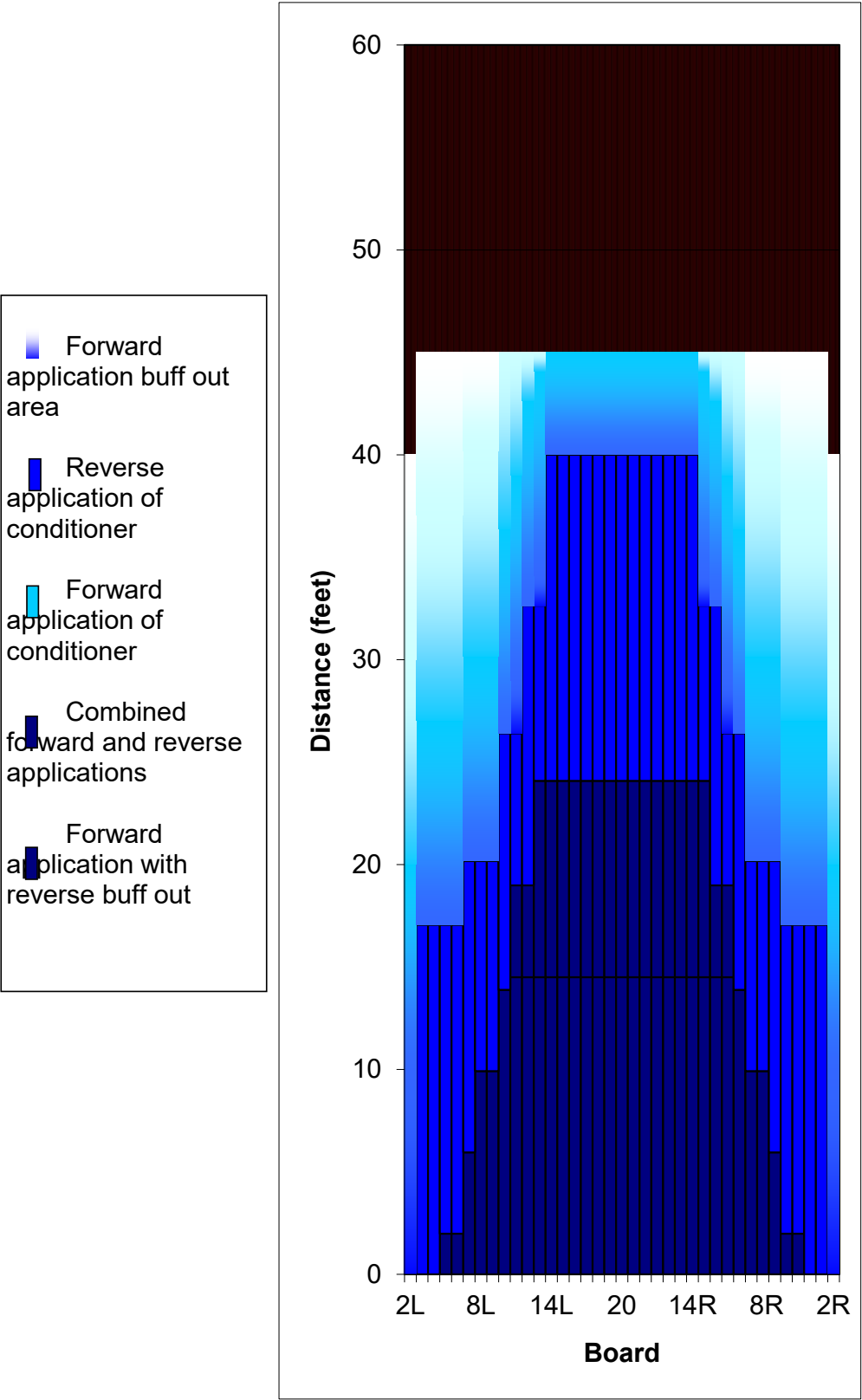
OB S ボウルレーンコンディション Overhead View of Conditioner Pattern
